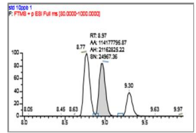
Sulfamethoxypridazin 磺胺甲氧吡嗪
