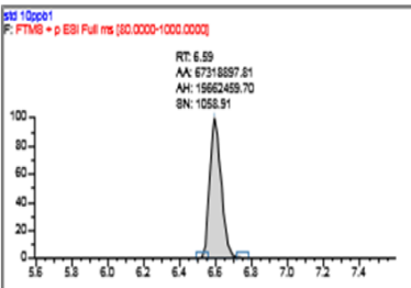
sulfisomidine 磺胺二甲异噻啉
