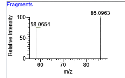
PROPIONYLPROMAZINE 丙酰丙嗪
