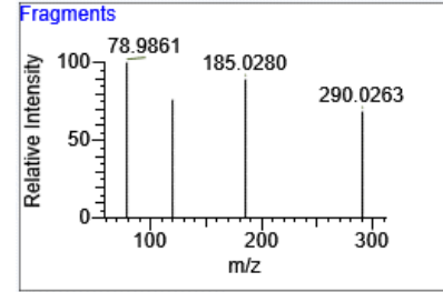
Thiamphenicol 甲砒霉素
