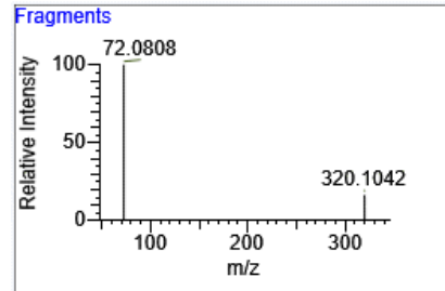
Marbofloxacin 马波沙星
