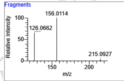
Sulfamethoxypridazin 磺胺甲氧吡嗪
