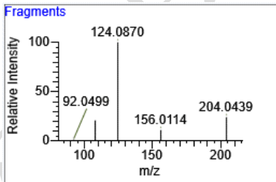
sulfisomidine 磺胺二甲异噻啉
