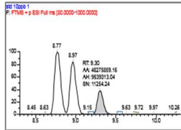
Sulfanomethoxine 磺胺间甲氧嘧啶
