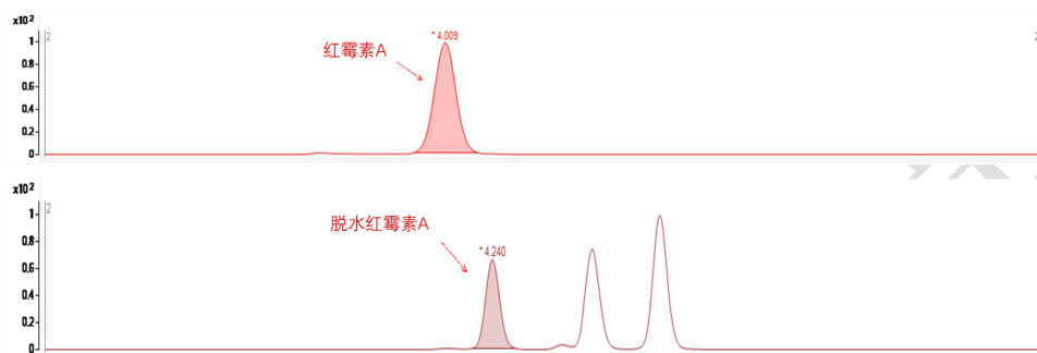
图 A.1 红霉素 A 及其降解物混合标准溶液 (10 \mu\text{g/L} ) 的 MRM 色谱图
