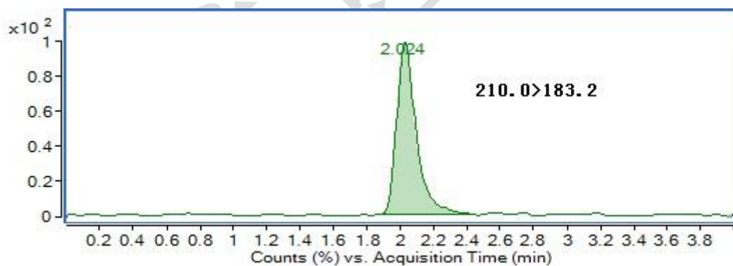
图 A.2 左旋咪唑-D 5 标准物质特征离子质量色谱图 (10 \mu\text{g/L} )
