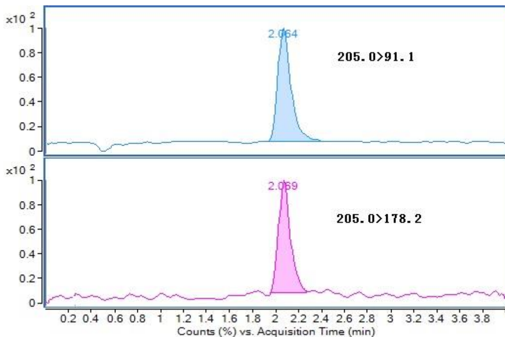
图 A.1 左旋咪唑标准物质特征离子质量色谱图 (2.5 \mu\text{g/L} )
